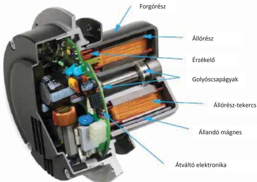
Energiatakarékos EC motor szerkezete
