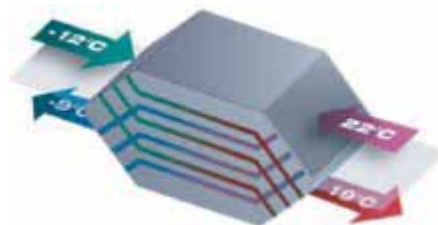
Ellenáramú, lemezes hőcserélő működési elve
